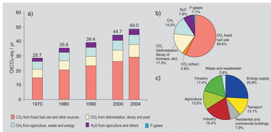
Figura 1 – Evolução da Emissão de Gases do Efeito Estufa - 1970-2004.
