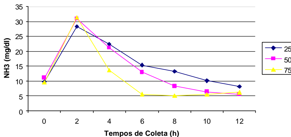
Figura 1. Concentrações ruminais de amônia (mg/dL), em diferentes tempos de amostragem, relacionadas com a proporção volumoso: concentrados da dieta (25:75, 50:50 e 75:25 de proporções volumoso: concentrados)
